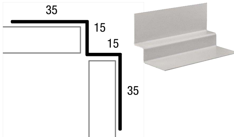
Внутренний угол
