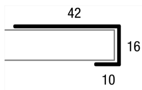
Соединительный профиль
