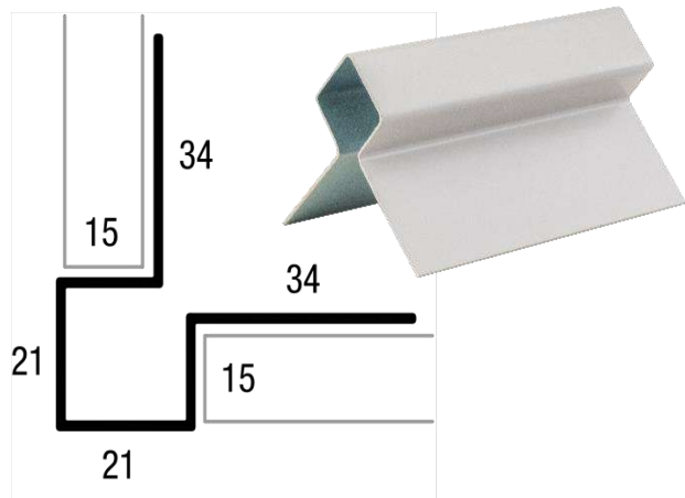
Внешний угол
